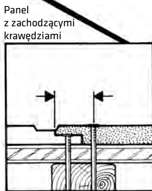
połączenie panelu
