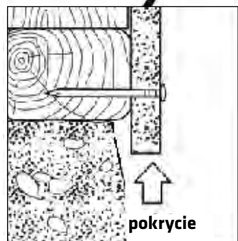
widok szczegółowy pasa dolnego
