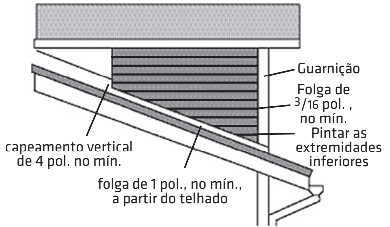
detalhe do capeamento do telhado
