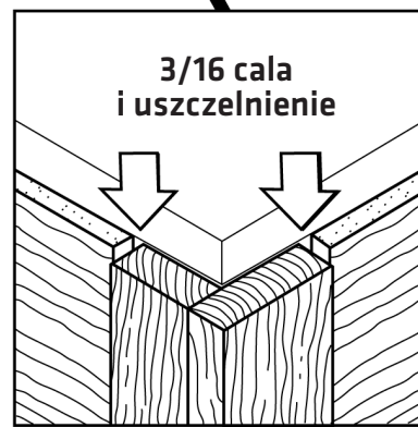
Widok szczegółowy narożnika zewnętrznego
